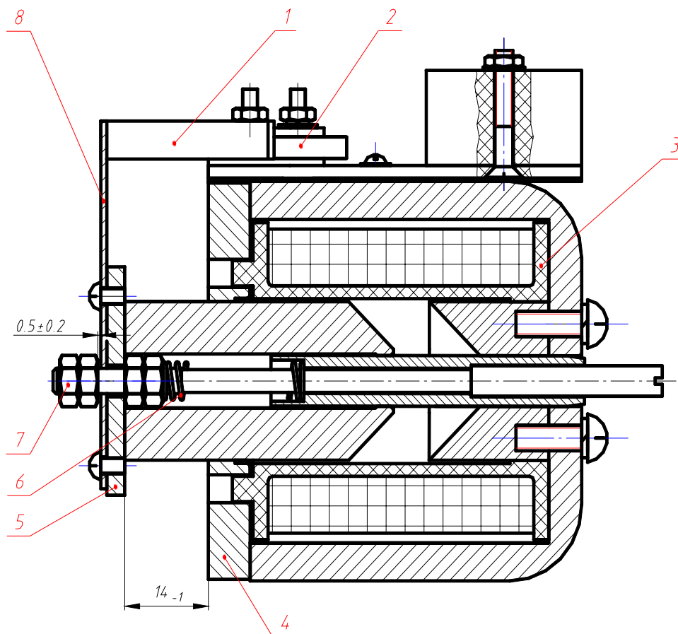
Рисунок 8 Расцепитель максимального тока
